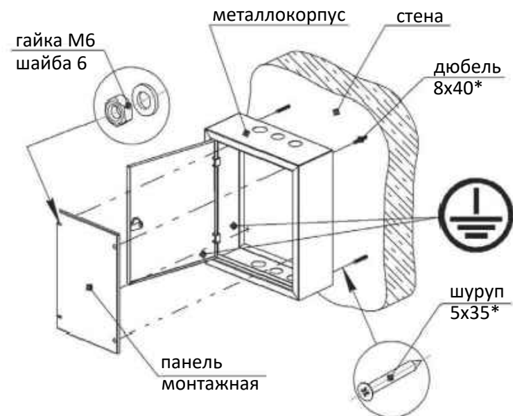
Рис.1. Схема монтажа
